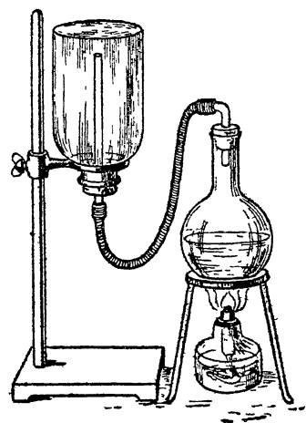
Рис. 40. Добывание аммиака.
