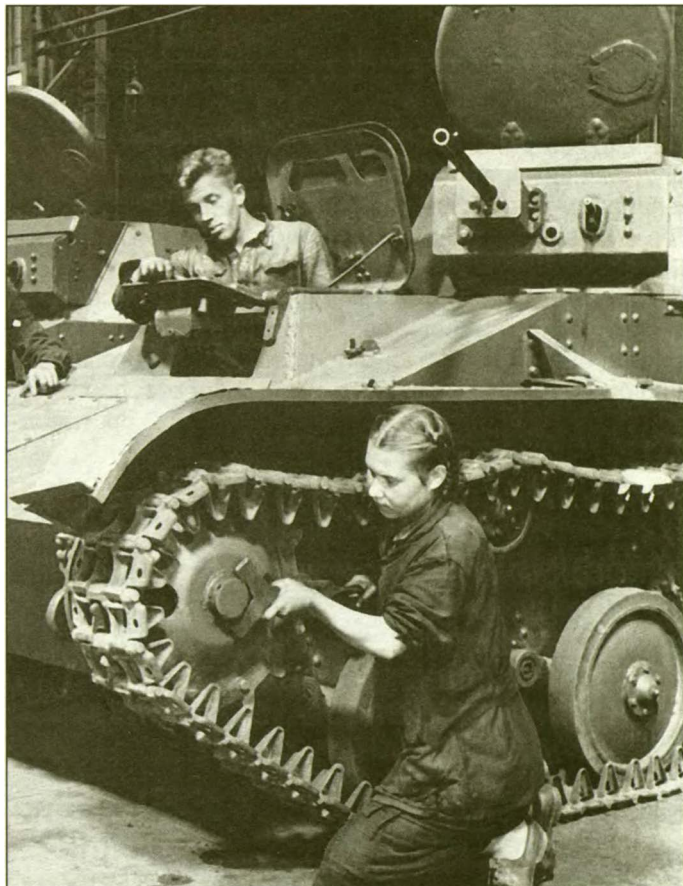
Ремонт танков на московском оборонном заводе. РГАКФД
