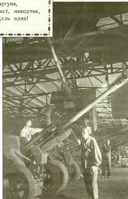
Цех артиллерийского вооружения. Москва. 1941 г. РГАКФД
